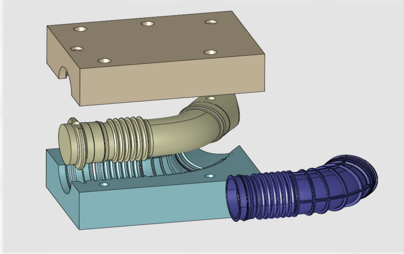
Kauçuk Hortum Kalıbı
