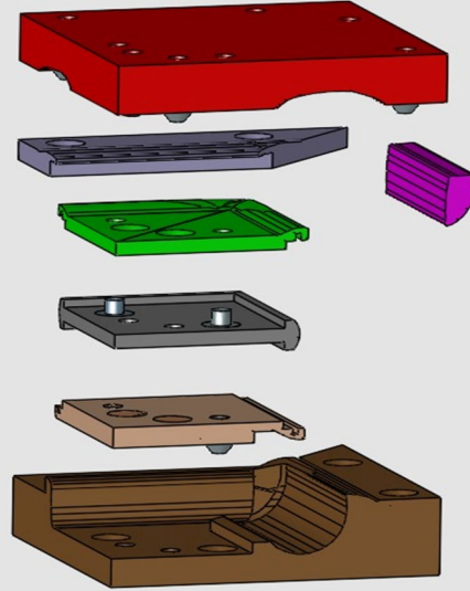
Köşe Kaynak Kalıbı
