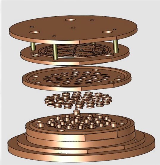
Kauçuk Enjeksiyon Kalıbı
