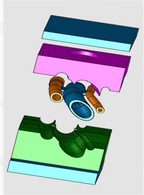
Hortum Birleştirme Kalıbı
