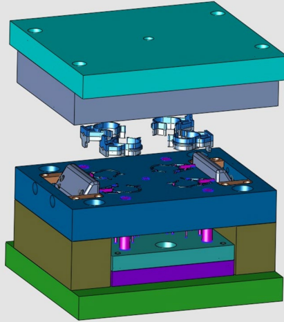
Klips Kalıbı
