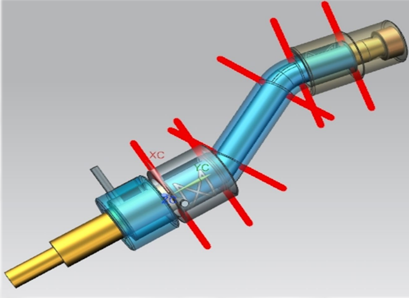
Çentikli Hareketli Burç Sistemi
