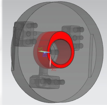
Profil Hortum Kalıbı
