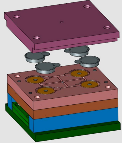
Tapa Kalıbı
