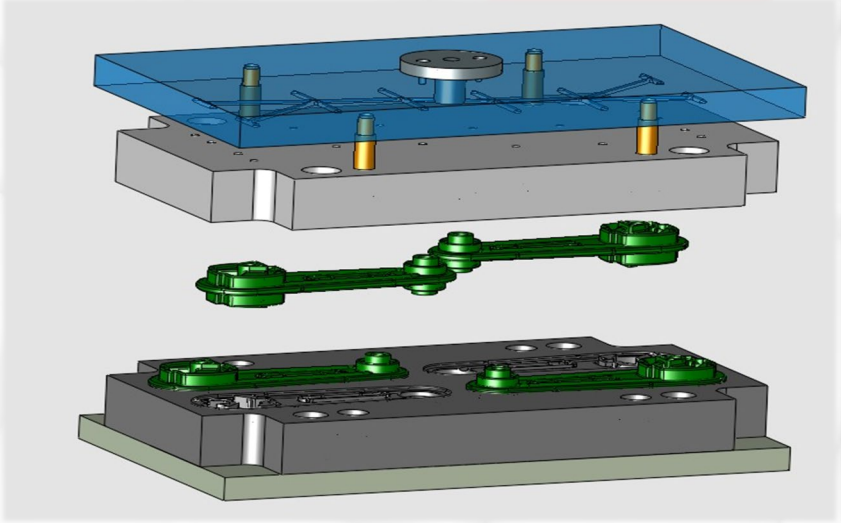
Kauçuk Overmold Kalıbı
